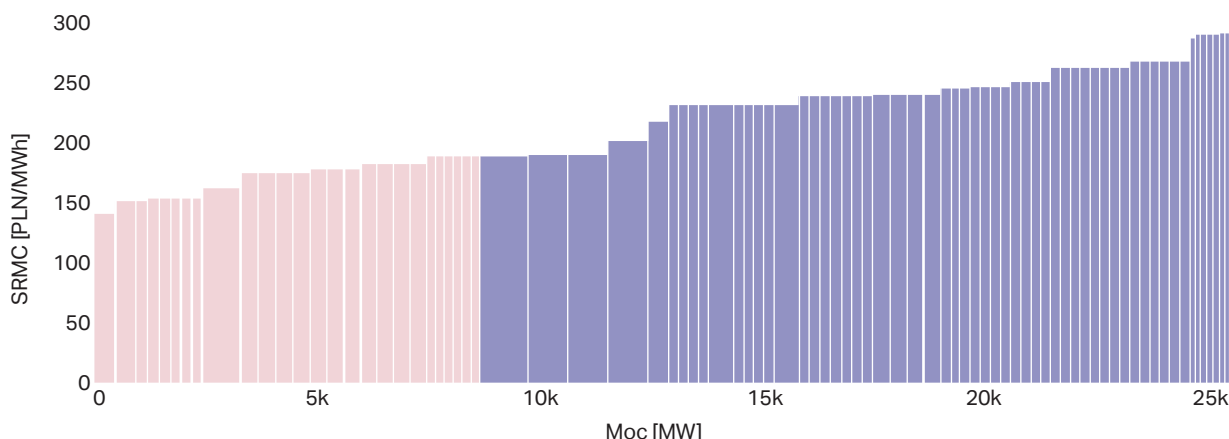
Rys. 5.2. Koszty zmienne wytwarzania energii elektrycznej w polskich elektrowniach węglowych (SRMC) w PLN/MWh
